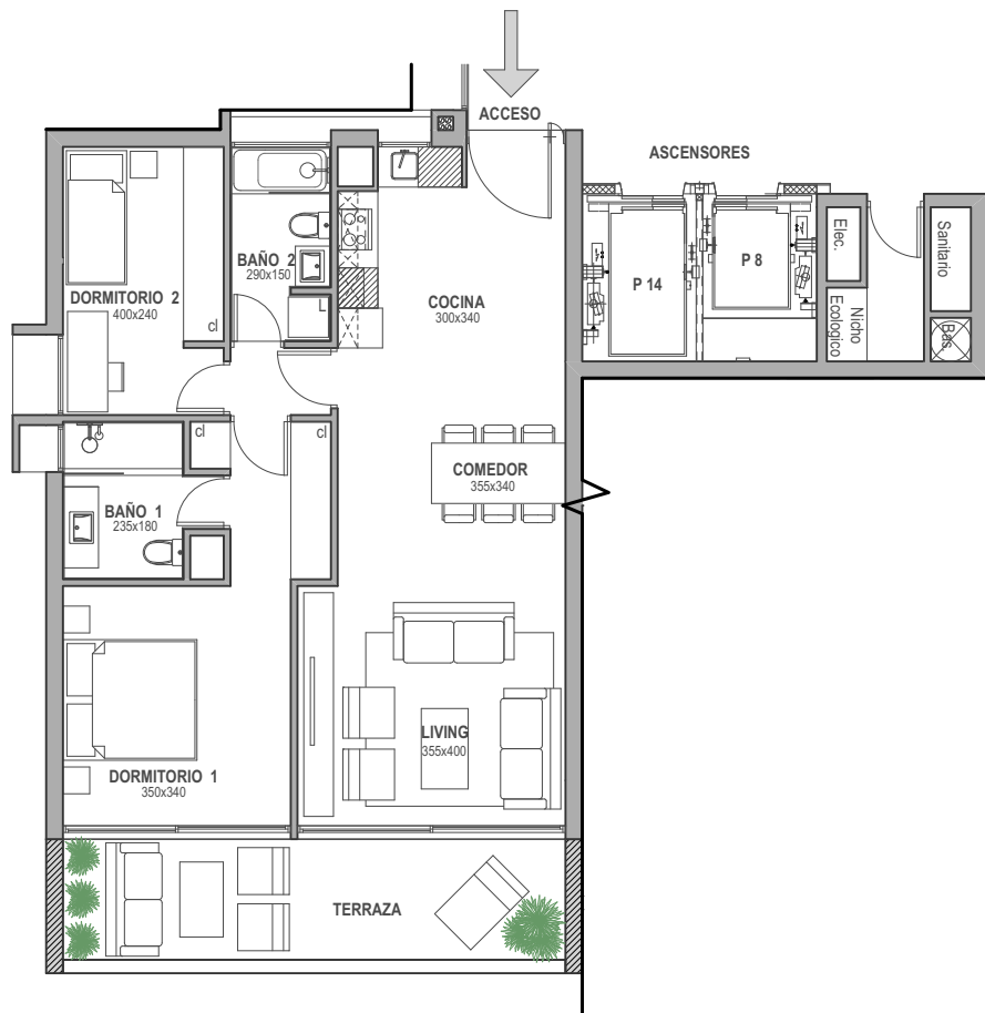
PLANTA ESC. 1:125
