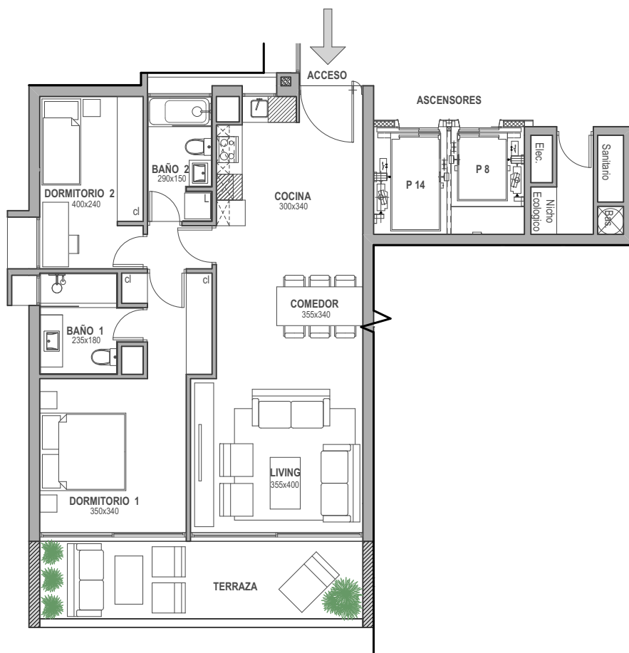
PLANTA ESC. 1:125
