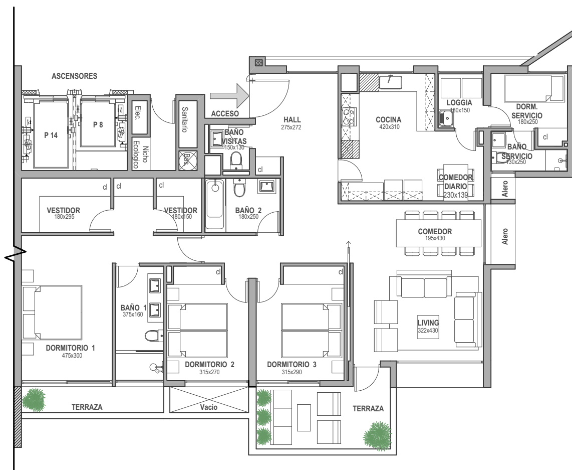
PLANTA ESC. 1:125
