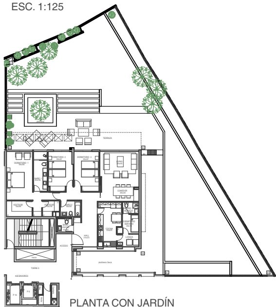
PLANTA ESC. 1:125
