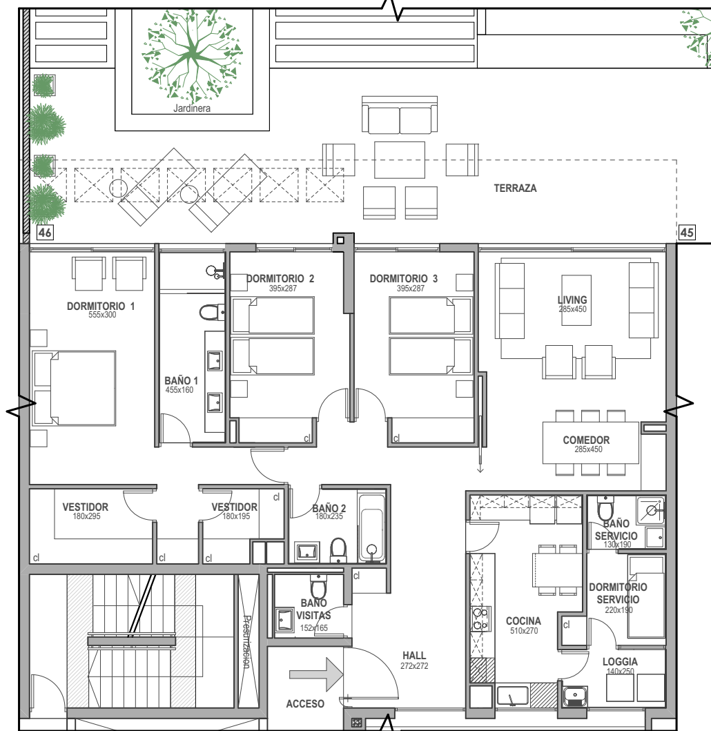
PLANTA ESC. 1:125
