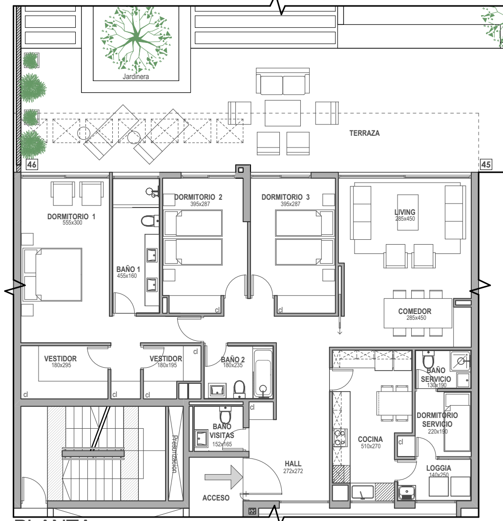
PLANTA ESC. 1:125
