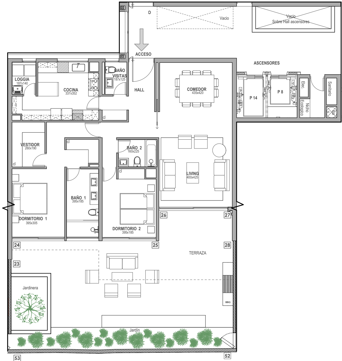
PLANTA ESC. 1:125
