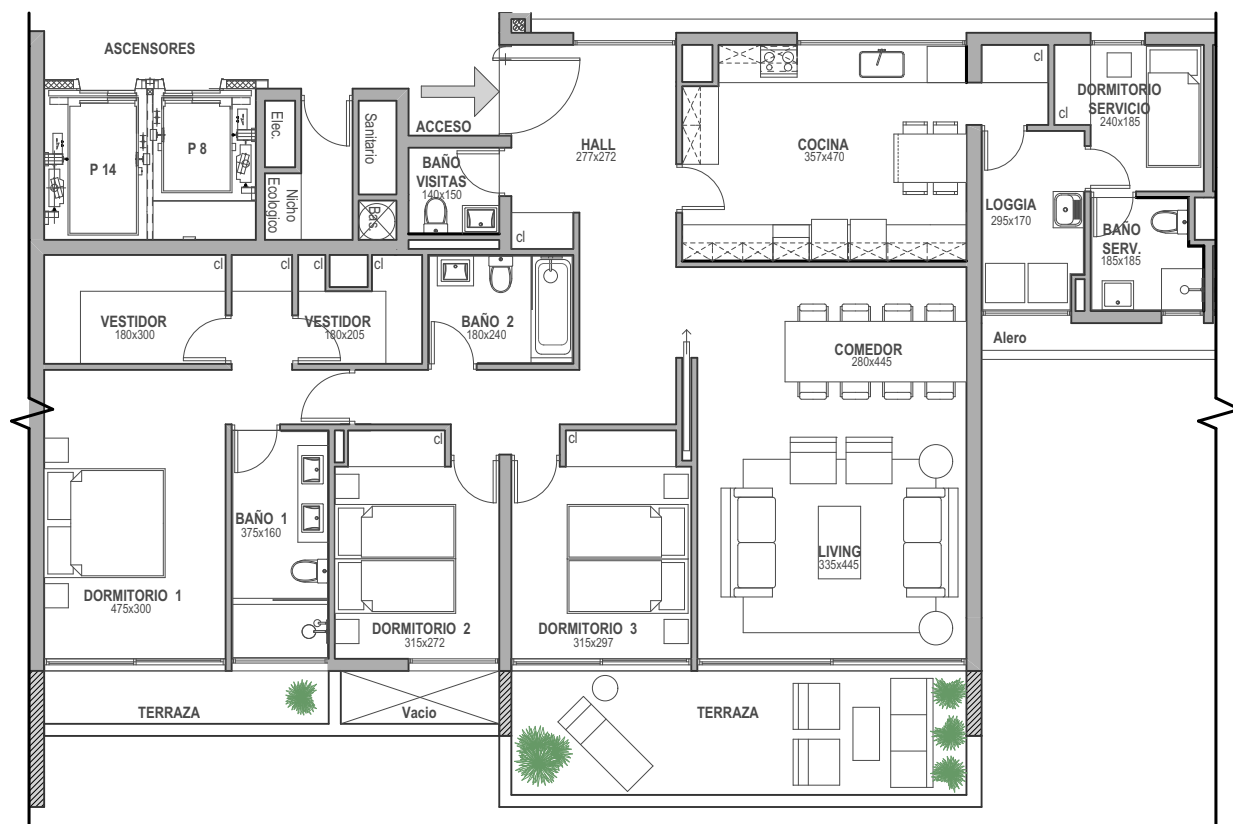
PLANTA ESC. 1:125
